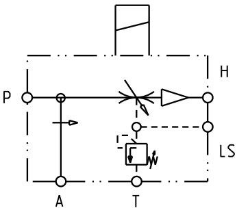
SCHEMA: A705-04D-G01
