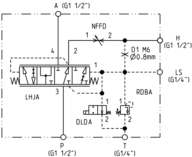
SCHEMA: A705-04D-G01
